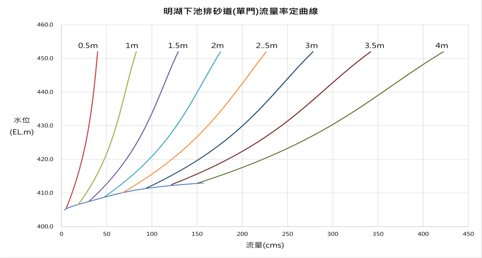
附圖二：排砂道閘門開度與水位、放流量關係圖
