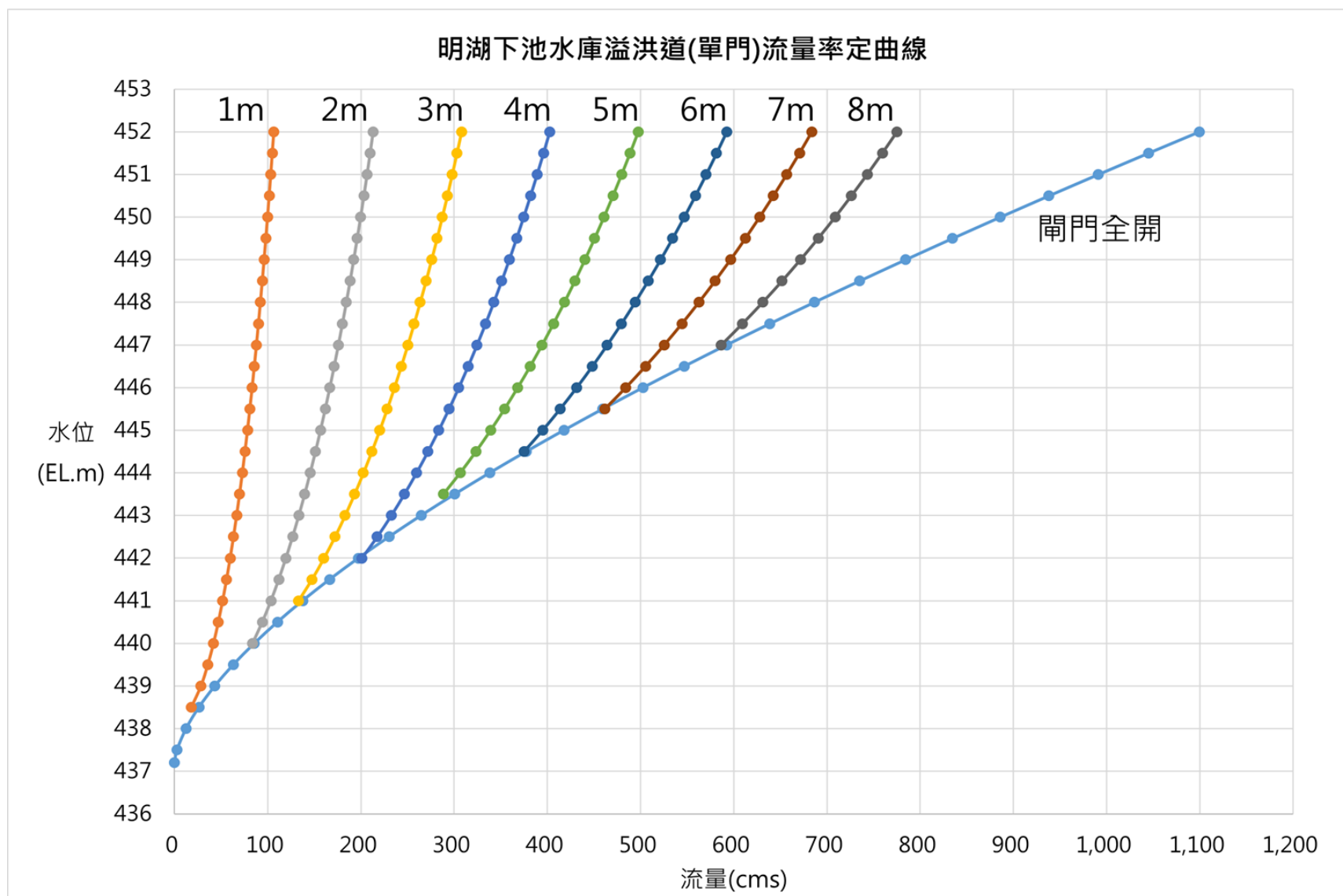
附圖一：溢洪道閘門開度與水位、放流量關係圖
